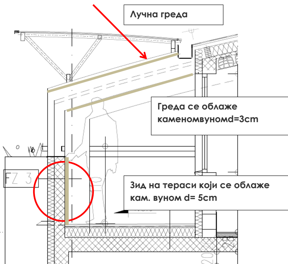
ЦРТЕЖ БР.2
